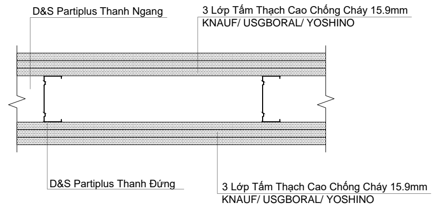
MẶT BẰNG
