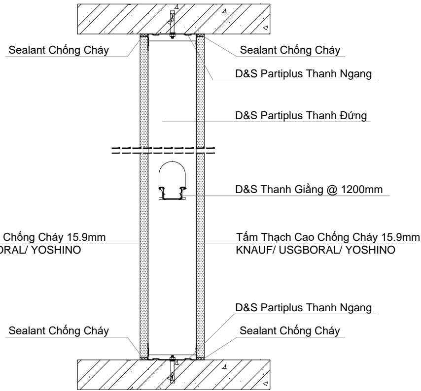
MẶT CẮT ĐỨNG
